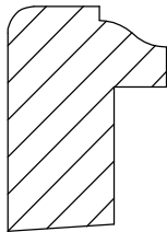
Backband 15-5 3/4" x 1 1/16"
