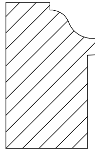
Backband 15-3 1" x 1 9/16"
